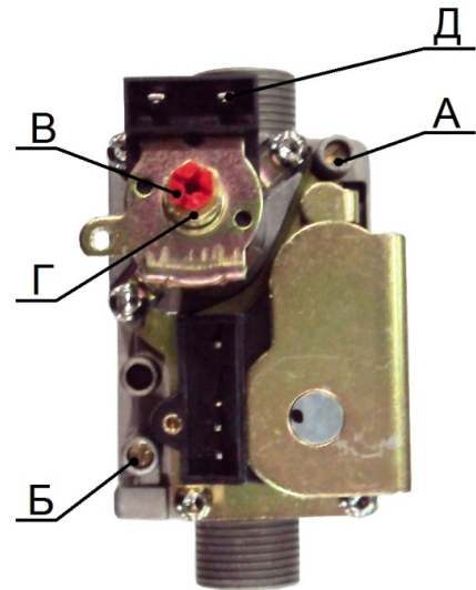
Рис. 6 Регулятор подачи газа
