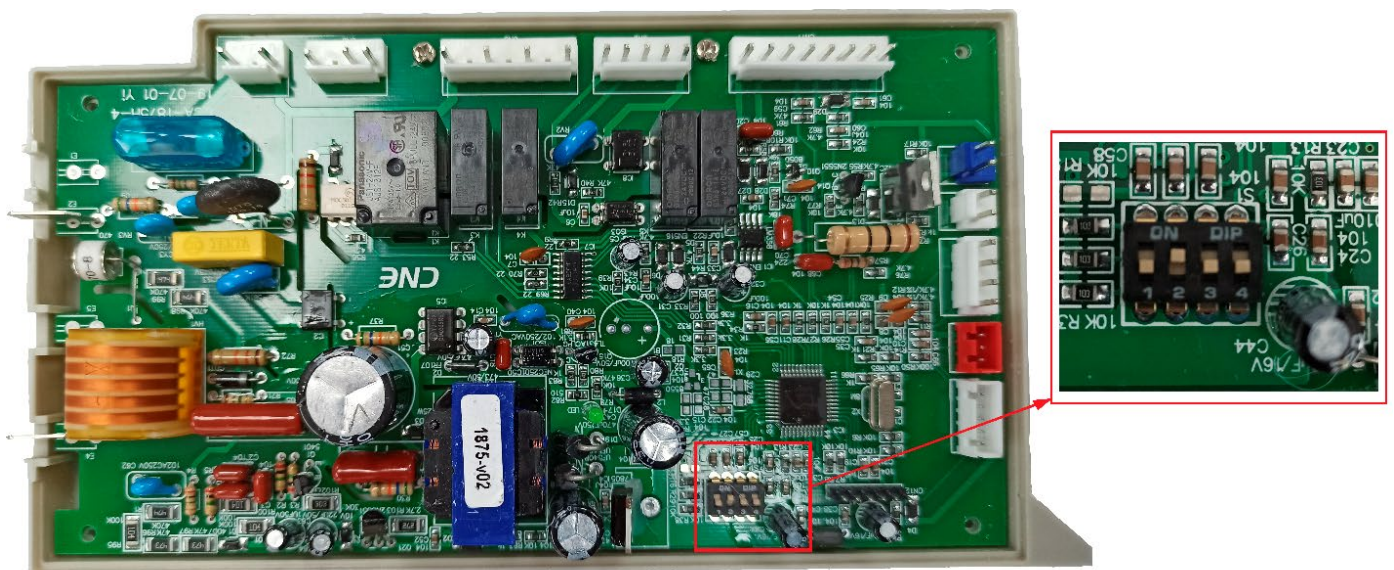
Рис. 7 Плата электронная и колодка переключателей
