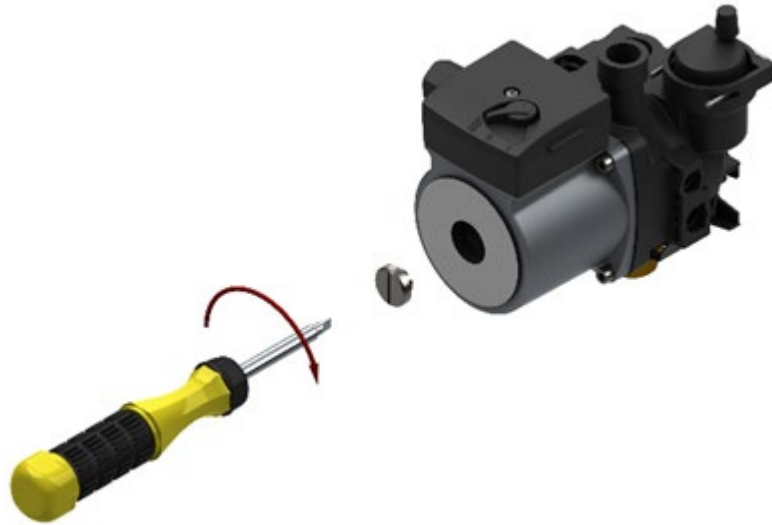
Рис. 5 Проверка циркуляционного насоса
